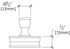
TOP VIEW SCALE: 6"=1'-0"
