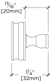
SIDE VIEW SCALE: 6"=1'-0"
