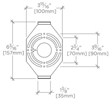
MOUNTING SCALE: 2"=1'-0"
