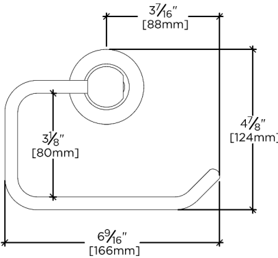
FRONT VIEW SCALE: 3"=1'-0"
