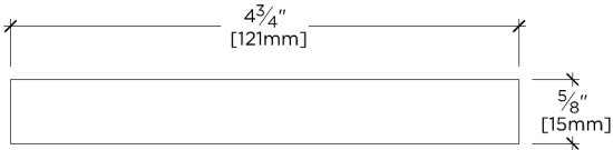
FRONT VIEW SCALE: 6"=1'-0"
