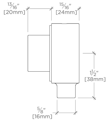
SIDE VIEW SCALE: 6"=1'-0"
