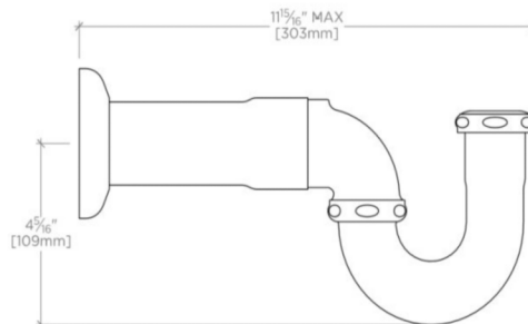
SIDE VIEW SCALE: 3"=1'-0"
