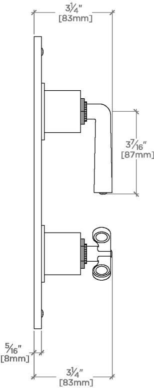
SIDE VIEW SCALE: 3"=1'-0"
