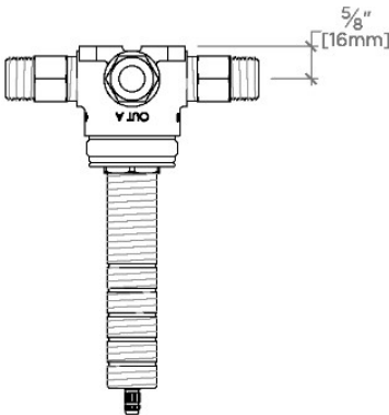
TOP VIEW SCALE: 3"=1'-0"
