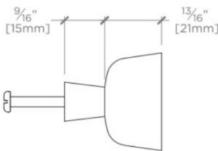
SIDE VIEW SCALE: 6"=1'-0"
