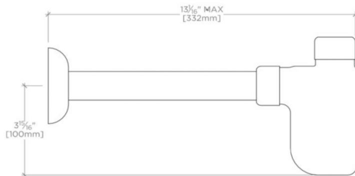
SIDE VIEW SCALE: 3"=1'-0"
