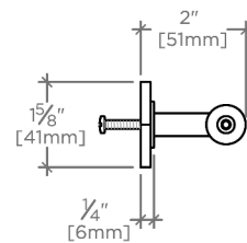
SIDE VIEW SCALE: 3"=1'-0"
