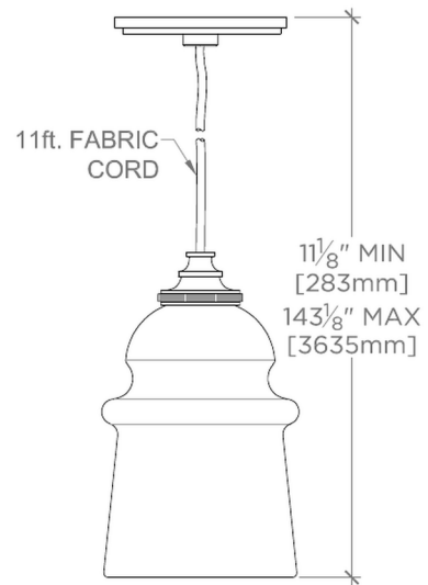
SIDE VIEW SCALE: 2"=1'-0"
