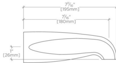
SIDE VIEW SCALE: 3"=1'-0"
