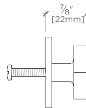
SIDE VIEW SCALE: 6"=1'-0"
