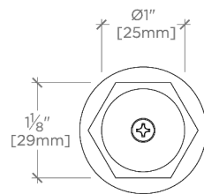
FRONT VIEW SCALE: 6"=1'-0"
