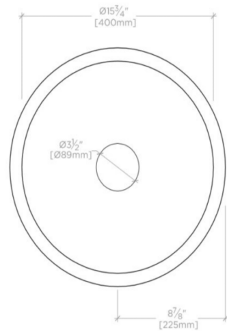
TOP VIEW SCALE: 1 1/2"=1'-0"
