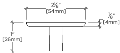
FRONT VIEW SCALE: 6"=1'-0"
