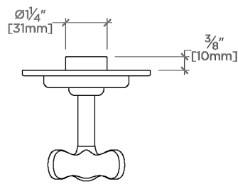
TOP VIEW SCALE: 3"=1'-0"
