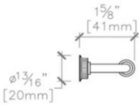
SIDE VIEW SCALE: 3"=1'-0"
