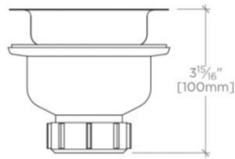
FRONT VIEW SCALE: 3"=1'-0"
