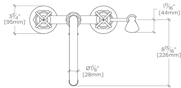
TOP VIEW SCALE: 1 1/2"=1'-0"
