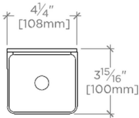
TOP VIEW SCALE: 1 1/2"=1'-0"
