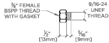
BSPP ADAPTER †
