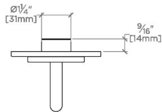
TOP VIEW SCALE: 3"=1'-0"
