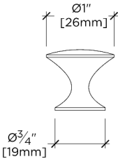
SIDE VIEW SCALE: 6"=1'-0"
