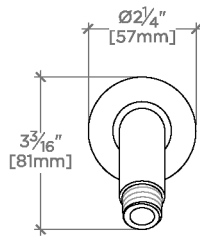
FRONT VIEW SCALE: 3"=1'-0"
