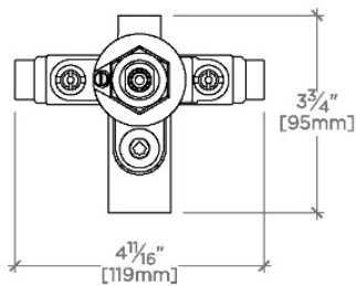
FRONT VIEW SCALE: 3"=1'-0"
