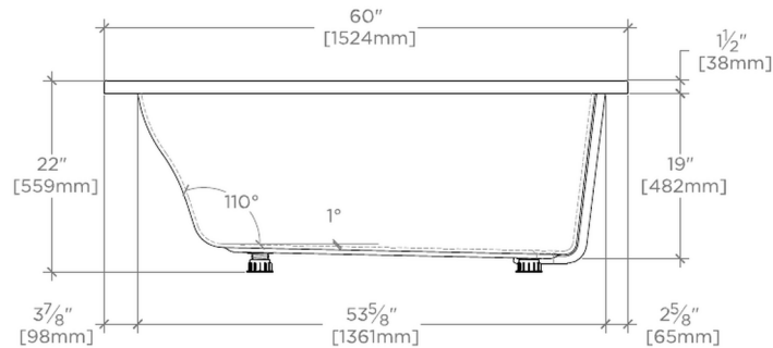
SCALE: 1/2"=1'-0"
