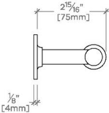
SIDE VIEW SCALE: 3"=1'-0"
