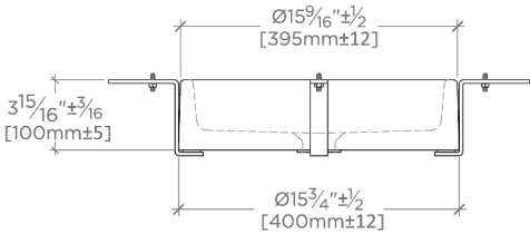
SIDE VIEW SCALE: 1"=1'-0"
