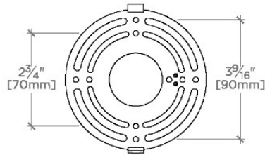
MOUNTING PLATE SCALE: 3"=1'-0"
