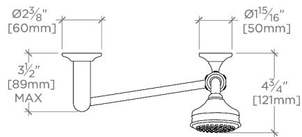
TOP VIEW SCALE: 1/2"=1'-0"
