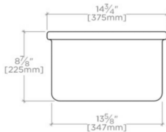
SIDE VIEW SCALE: 1"=1'-0"
