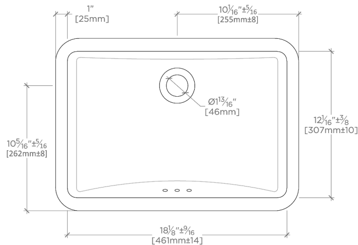
TOP VIEW SCALE: 1 1/2"=1'-0"
