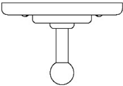
TOP VIEW SCALE: 3"=1'-0"
