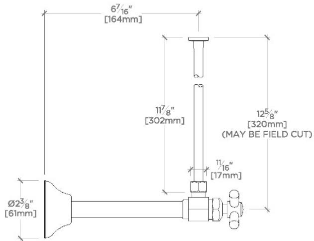
SIDE VIEW SCALE: 3"=1'-0"
