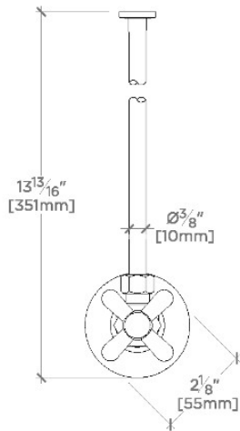
FRONT VIEW SCALE: 3"=1'-0"
