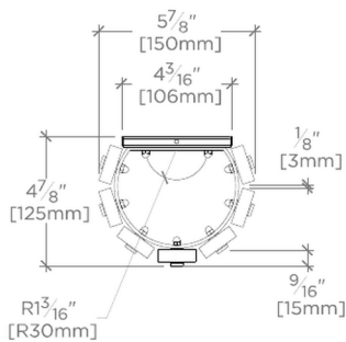
TOP VIEW SCALE: 1 1/2"=1'-0"
