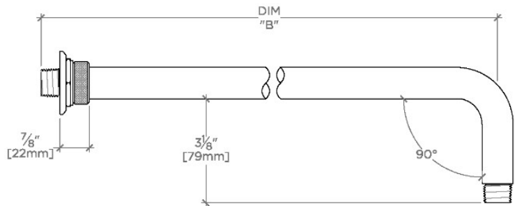
SIDE VIEW SCALE: 3"=1'-0"
