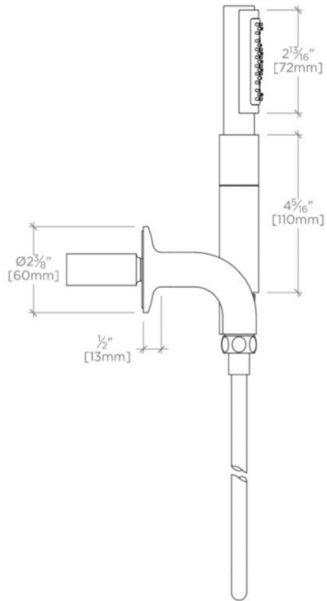
SIDE VIEW SCALE: 3"=1'-0"
