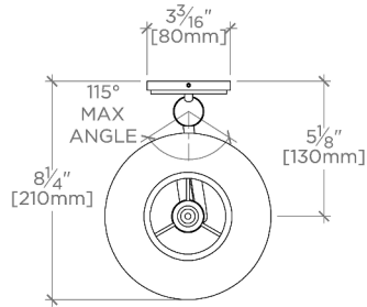
TOP VIEW SCALE: 1\frac{1}{2}"=1'-0"
