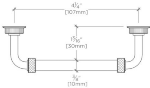
TOP VIEW SCALE: 6"=1'-0"
