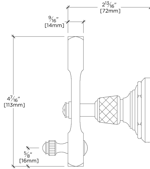
SIDE VIEW SCALE: 6"=1'-0"
