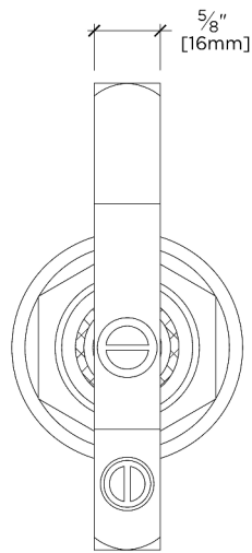
FRONT VIEW SCALE: 6"=1'-0"
