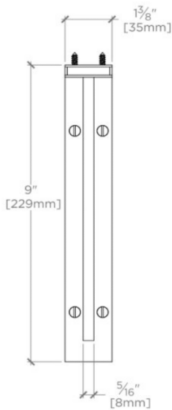
FRONT VIEW SCALE: 3"=1'-0"
