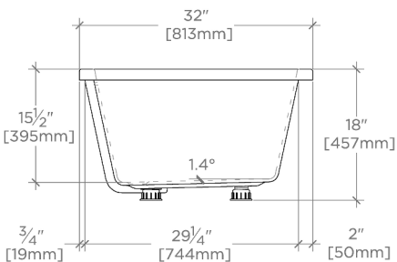
END VIEW SCALE: 1/2"=1'-0"
