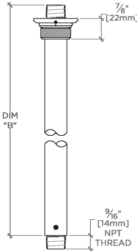
SIDE VIEW SCALE: 3"=1'-0"
