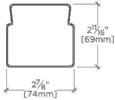
FRONT VIEW SCALE: 3"=1'-0"
