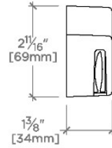
SIDE VIEW SCALE: 3"=1'-0"
