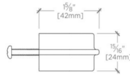
SIDE VIEW SCALE: 6"=1'-0"
