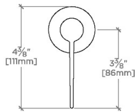
FRONT VIEW SCALE: 3"=1'-0"
