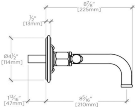
SIDE VIEW SCALE: 2"=1'-0"
