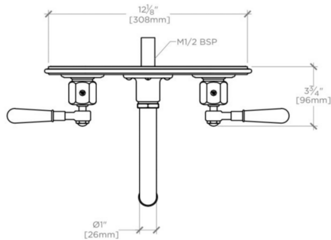
TOP VIEW SCALE: 2"=1'-0"
