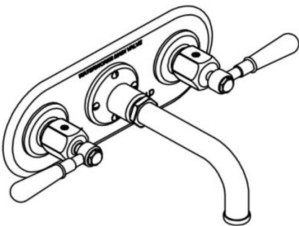
ISO VIEW SCALE: 2"=1'-0"
