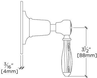
SIDE VIEW SCALE: 3"=1'-0"
