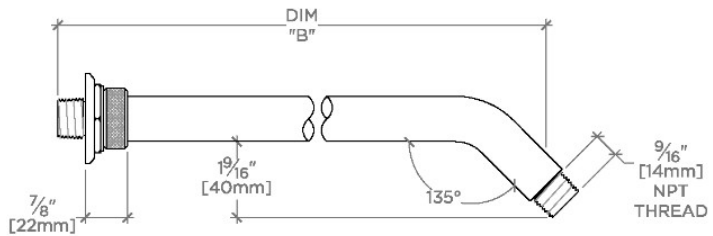
SIDE VIEW SCALE: 3"=1'-0"
